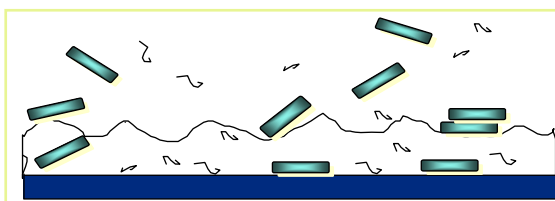
Фиг.1. Схема на „закрепване“ и действие на микроорганизмите и ензимите
